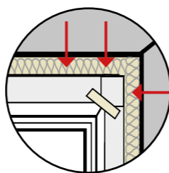
Fuge umlaufend hohlraumfrei mit Dämmstoff ausfüllen
