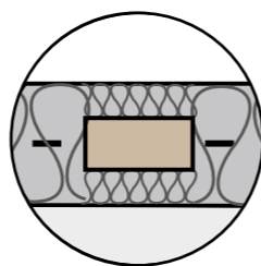
Tragklotz überdämmen
